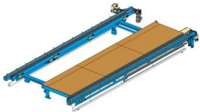
Stół do zbijania szkieletów FT2000
