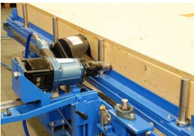
Widok ogólny stacji Double System – SF021.
