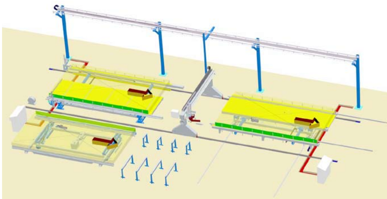
Widok stacji Double System, stacji z serii Flexi
