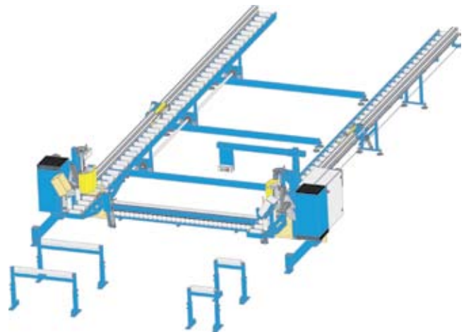
Stacja do zbijania szkieletów FM1000TS
