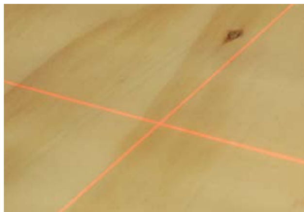
Widok przedstawiający marker laserowy NB1-LF montowany na moście zbijającym NB1000 zapewniający łatwe i precyzyjne ustawienia podczas operacji zbijania, pitowania lub frezowania.
