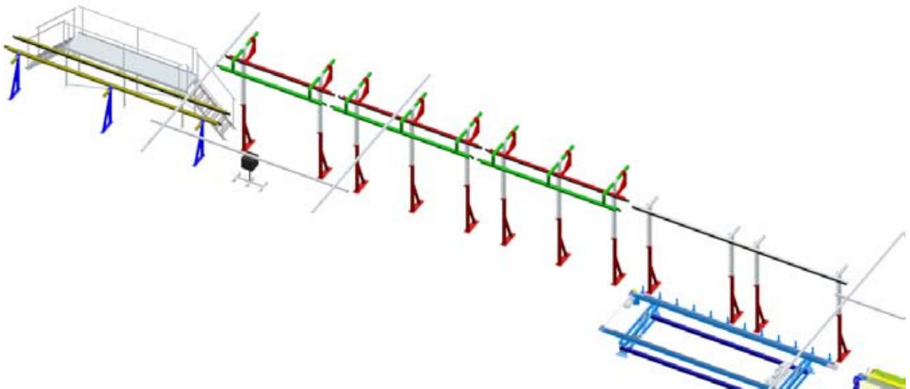
Widok przedstawiający kompletny przenośnik wyjściowy elementów w pozycji pionowej, który można integrować z wszystkimi systemami z serii Flexi.
